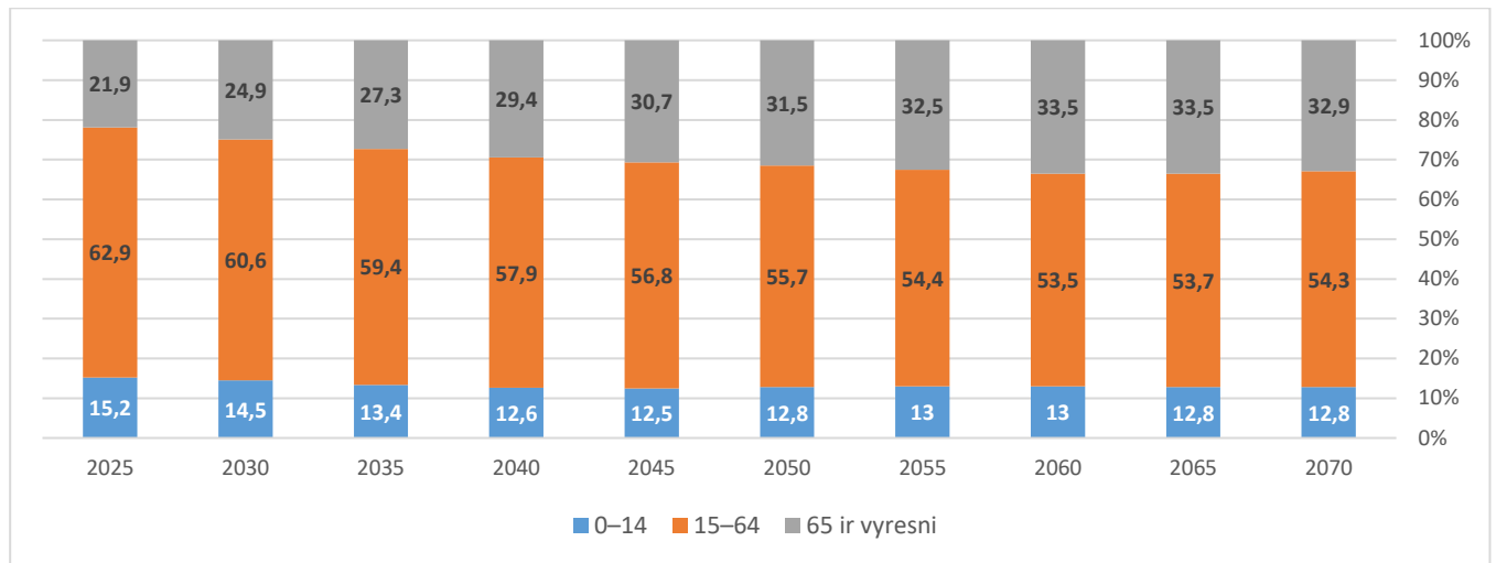
6 pav. Gyventojų struktūros šalyje pagal amžiaus grupes prognozė iki 2070 m.
