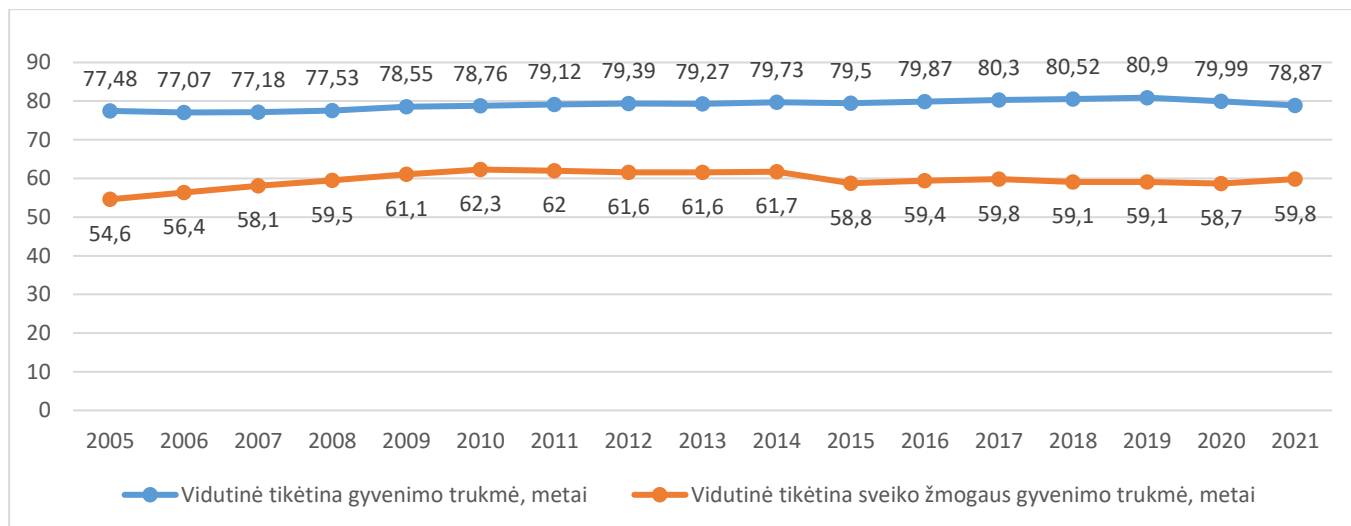
4 pav. Vidutinė tikėtina gyvenimo trukmė, 0 m. amžiaus moterų, šalyje
